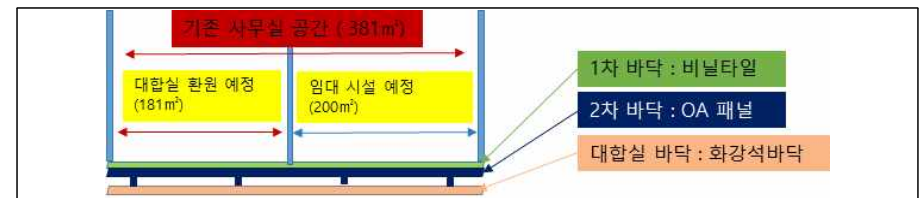
【표】 터미널 내부 리모델링 공사 바닥면 단면도
