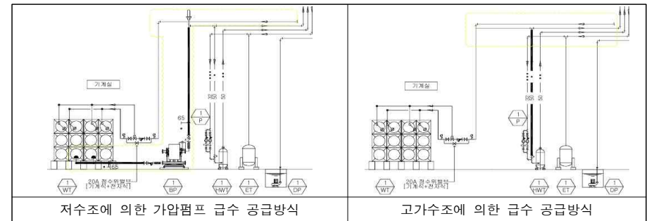
【표2】급수 공급방식 변경 계통도
